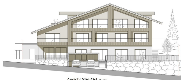
Ansicht Süd-Ost M:1:100
