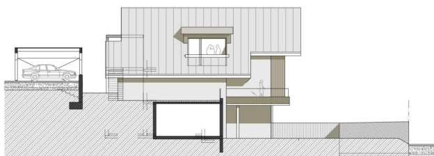
Schnittansicht B-B Süd-West M:1:100
